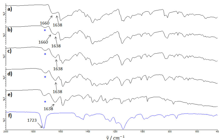
Slika 8.54: IR spektri praćenja ILAG reakcije L2 i \text{PdCl}_2 s \text{NaOAc} (u množinskom omjeru 1:4:2) i 15 \mu\text{L} DMF nakon: a) 15 min, b) 45 min, c) 90, d) 2 h, e) 4 h i f) PMMA, materijal od kojeg je izrađena reakcijska posuda. Vrpca pri 1723 \text{cm}^{-1} po kojoj određena prisutnost PMMA u reakcijskim smjesama označena je plavom zvjezdicom.
