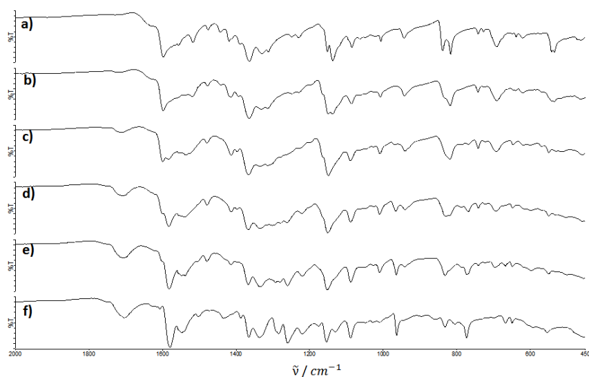
Slika 8.53: IR spektri ^1 IAG reakcije L2 i \text{PdCl}_2 s \text{NaOAc} kao aditivom u množinskom omjeru 1:4:2 nakon: a) 15 min, b) 30 min, c) 1 h, d) 2 h, e) 4 h i f) 6 h. Reakcijske smjese sadrže malu količinu PMMA od kojeg je izrađena reakcijska posuda, a kojem je pripisana vrpca pri 1723 \text{cm}^{-1} .
