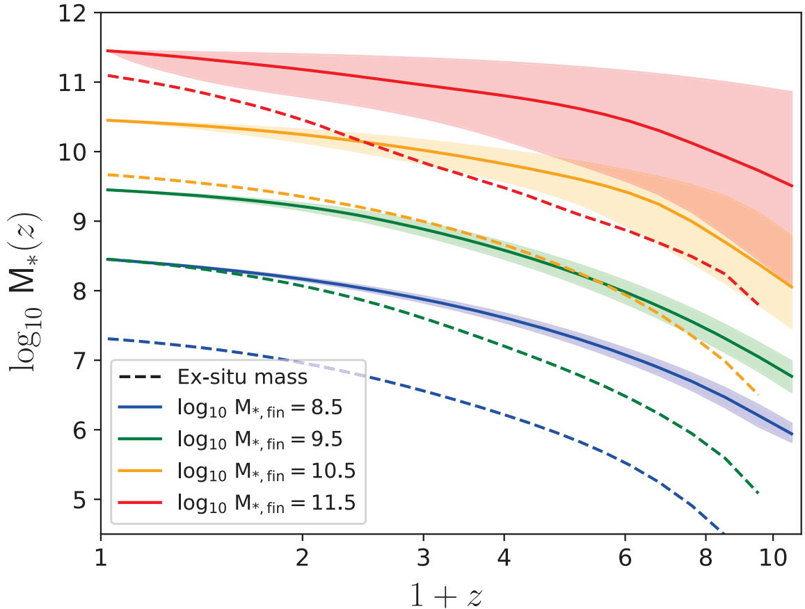
Slika 4.15: Evolucija zvjezdane mase galaksija za par konačnih zvjezdanih masa (prema legendi). Evolucija je računata preko jednađbe (4.14). Zasjenjena područja predstavljaju pouzdanost u srednjem rezultatu.
