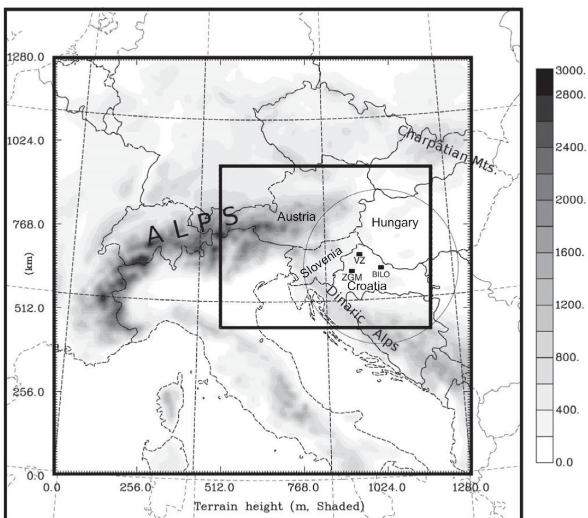
Slika 26 Domene tri ARPS konfiguracije: ARPS24 (horizontalni korak mreže 24 km) – najveći četverokut, ARPS8 (horizontalni korak mreže 8 km) – srednji četverokut i ARPS2.5 (horizontalni korak mreže 2.5 km) – najmanji četverokut. Prikazane su i lokacije radiosondažane postaje Zagreb Maksimir (ZGM), grada Varaždina (VZ) i radarske postaje RC Biloga (BILO). Kružnica sa središtem u lokaciji BILO predstavlja maksimalni domet radara (240 km).
