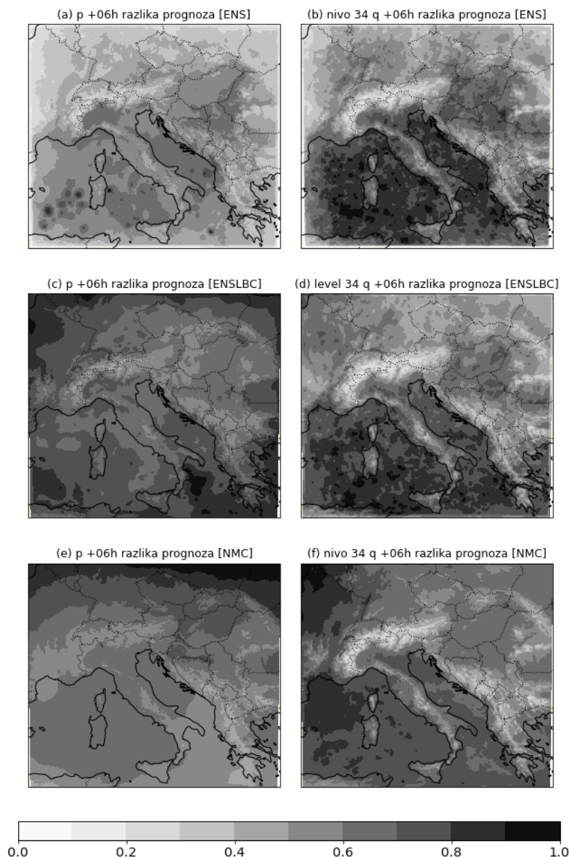
Slika 10 Normalizirane standardne devijacije površinskog tlaka za: (a) ENS, (c) ENSLBC i (e) NMC eksperiment. Normalizirane standardne devijacije specifične vlažnosti na 34. nivou modela (otprilike 500 hPa) za (b) ENS, (d) ENSLBC i (f) NMC eksperiment. Normalizacija je provedena dijeljenjem standardnih devijacija s maksimalnom horizontalnom vrijednosti standardne devijacije za promatranu varijablu. Maksimalne vrijednosti standardnih devijacija za površinski tlak su: ENS: 0.6 hPa; ENSLBC: 0.77 hPa; NMC: 6.67 hPa. Maksimalne vrijednosti standardnih devijacija za specifičnu vlažnost na 34. nivou modela su: ENS: 0.26 g/kg, ENSLBC: 0.29 g/kg; NMC: 0.55 g/kg.
