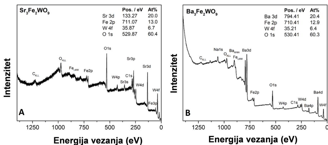
Slika 52. XPS-spektri spojeva \text{Sr}_3\text{Fe}_2\text{WO}_9 (lijevo) i \text{Ba}_3\text{Fe}_2\text{WO}_9 (desno) snimljeni u širokom području energija vezanja.
