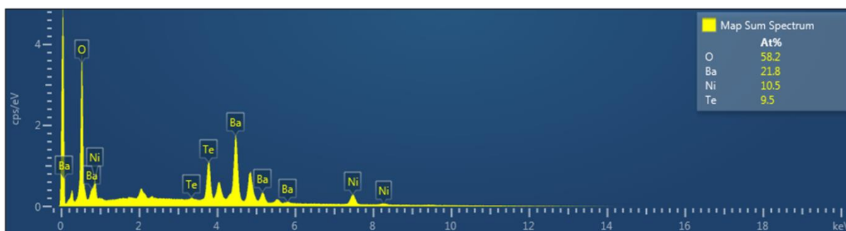
Slika D12. EDX spektar BNTO.
