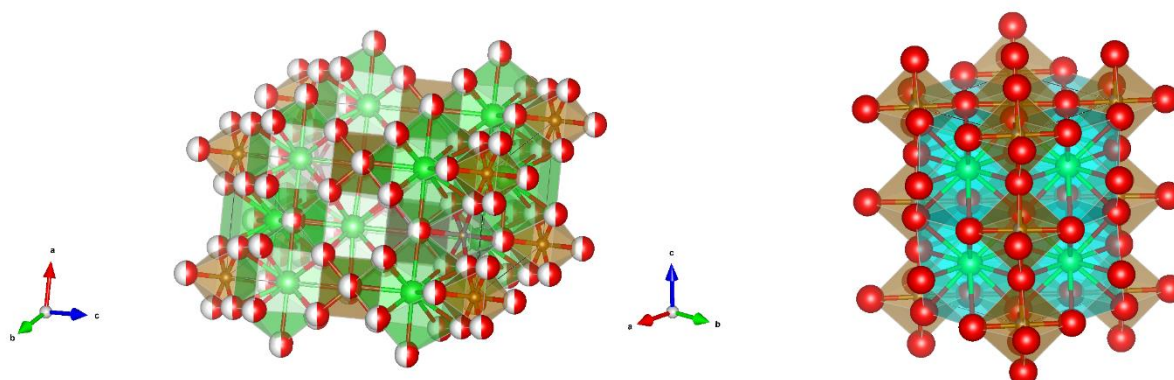
Slika 41. Struktura heksagonskog \text{Ba}_3\text{Fe}_2\text{WO}_9 (lijevo) i tetragonskog \text{Sr}_3\text{Fe}_2\text{WO}_9 (desno).
