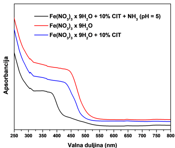
Slika 34. Apsorpcijski UV/Vis-spektar vodene otopine željezovog(III) nitrata nonahidrata, c = 1 \cdot 10^{-3} \text{ mol dm}^{-3} (crveno), željezovog(III) nitrata nonahidrata u 10%-tojoj vodenoj otopini limunske kiseline (plavo) i željezovog(III) nitrata nonahidrata u 10%-tojoj vodenoj otopini limunske kiseline uz dodatak koncentrirane otopine amonijaka, \text{pH} = 5 (crno).
