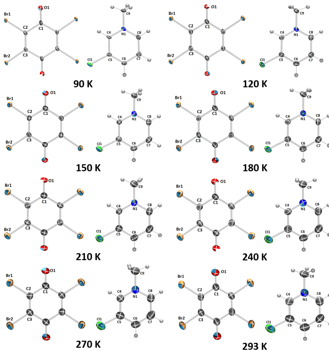
Slika D4. Prikaz elipsoida pomaka radikal-aniona \text{Br}_4\text{Q}^- (lijevo) i kationa N\text{-Me-3-Clpy}^+ (desno) u spoju 4 (vjerojatnost nalaženja 50 %) pri različitim temperaturama, 90–293 K.
