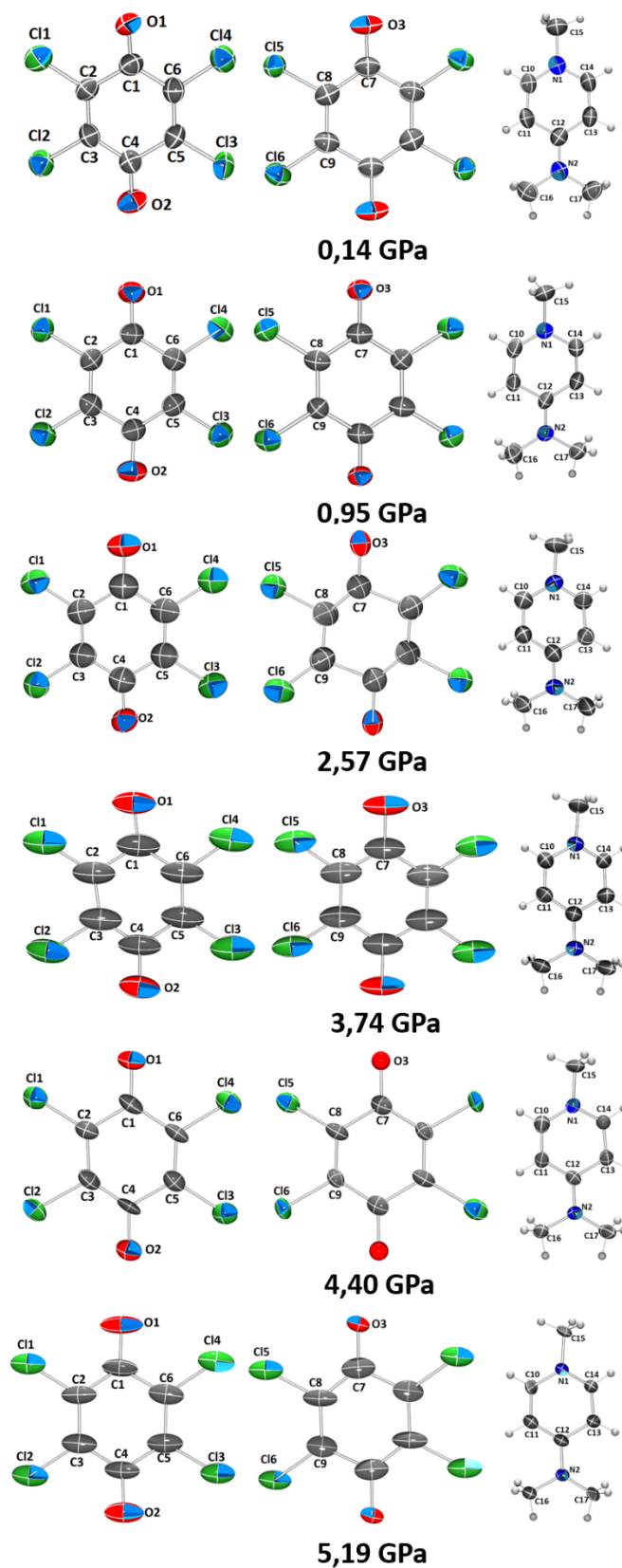
Slika D6. Prikaz elipsoida pomaka radikal-aniona \text{Cl}_4\text{Q}^{\bullet-} (lijevo) i kationa 4\text{-damp}^+ (desno) u spoju 2 (vjerojatnost nalaženja 50 %) pri visokom tlaku od 0,14–5,19 GPa.
