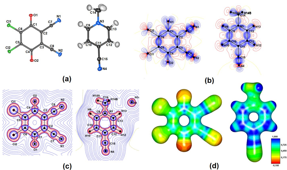
Slika 37. Molekulska struktura radikal-aniona \text{DDQ}^- (lijevo) i kationa N\text{-Me-4-CNpy}^+ (desno): (a) prikaz elipsoida pomaka (vjerojatnost nalaženja 70 %), (b) mape deformacijske gustoće (konture 0,05 e \text{Å}^{-3} ), (c) mape laplasijana (konture 2, 4, 8 \cdot 10^n e \text{Å}^{-5} , n=3 \cdots 2 ) i d) elektrostatski potencijal mapiran na izopovršinu elektronske gustoće 0,5 e \text{Å}^{-3} .
