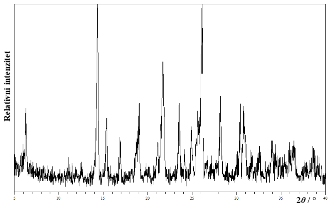
Slika D33. Difraktogram praškastog uzorka samljevene smjese o:13fib = 1 : 1.
