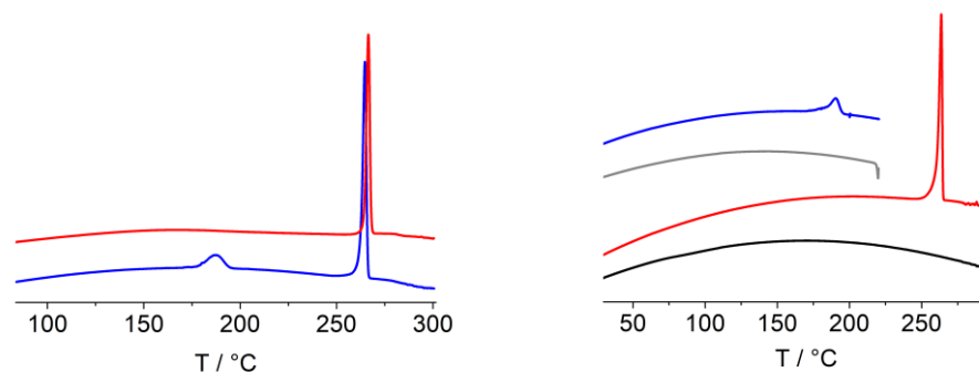
Slika 46. DSC termogrammi ciklusa grijanja B1az zn ( mer , crveni) i B1b zn ( fac , plava), lijevo. Temperaturno kontrolirani prijelaz polimorfa fac u mer , desno.
