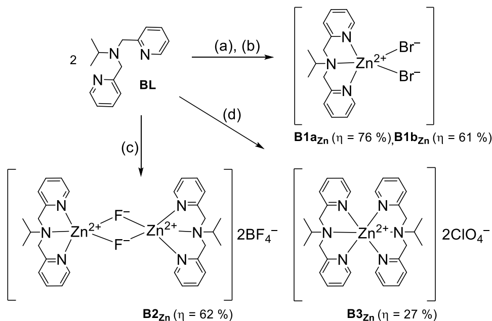
Slika 43. Sinteza Zn(II) kompleksa liganda BL . Reakcijski uvjeti: (a) \text{ZnBr}_2 , metanol; (b) 2 \text{ZnBr}_2 , 4 \text{NH}_4\text{PF}_6 , metanol, (c) \text{Zn}(\text{BF}_4)_2 , metanol; (d) \text{Zn}(\text{ClO}_4)_2 , metanol, kloroform.
