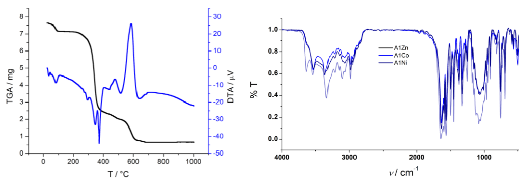
Slika 30. Termogram A1 Zn (lijevo) i usporedba IR spektara kompleksa A1 Zn , A1 Co i A1 Ni (desno).
