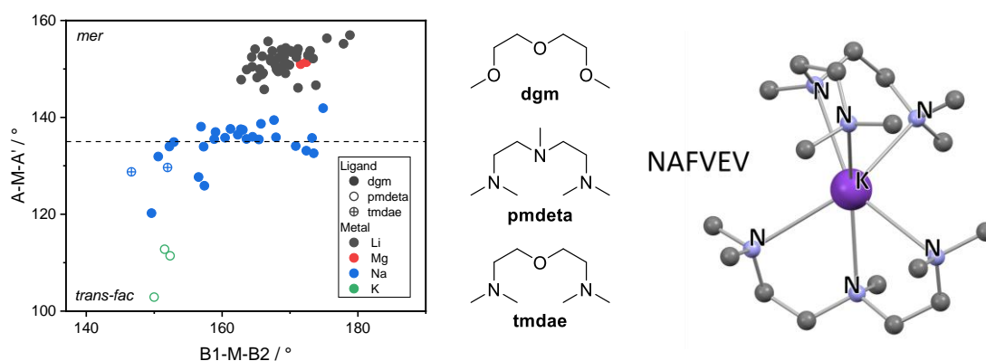
Slika 9. Ovisnost A-M-A' o B1-M-B2 kutovima za 74 [M(\mathbf{dgm})_2] kompleksa s ligandima dgm , pmdeta , i tmdae . Deformirana koordinacijska geometrija [K(\mathbf{pmdeta})_2]^+ kompleksnog kationa NAFVEV.
