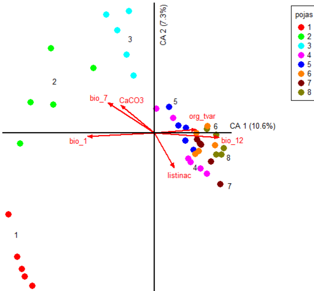
Slika 117 Ordinacijski graf CCA analize vegetacijskih snimki ukupne flore duž visinskog transeka Sjevernog Velebita (bio_1 – srednja godišnja temperatura, bio_7 – godišnji raspon temperatura, bio_12 – godišnja precipitacija; 1 – pojas hrasta crnike, 2 – pojas bijelog graba, 3 – pojas crnog grba, 4 – pojas primorske bukve, 5 – pojas bukve i jele, 6 – pojas smreke, 7 – pojas pretplaninske bukve i 8 – pojas bora krivulja) (vlastita vrijednost ( eigenvalue ) za prvu os iznosi 0,787, za drugu os 0,543)
