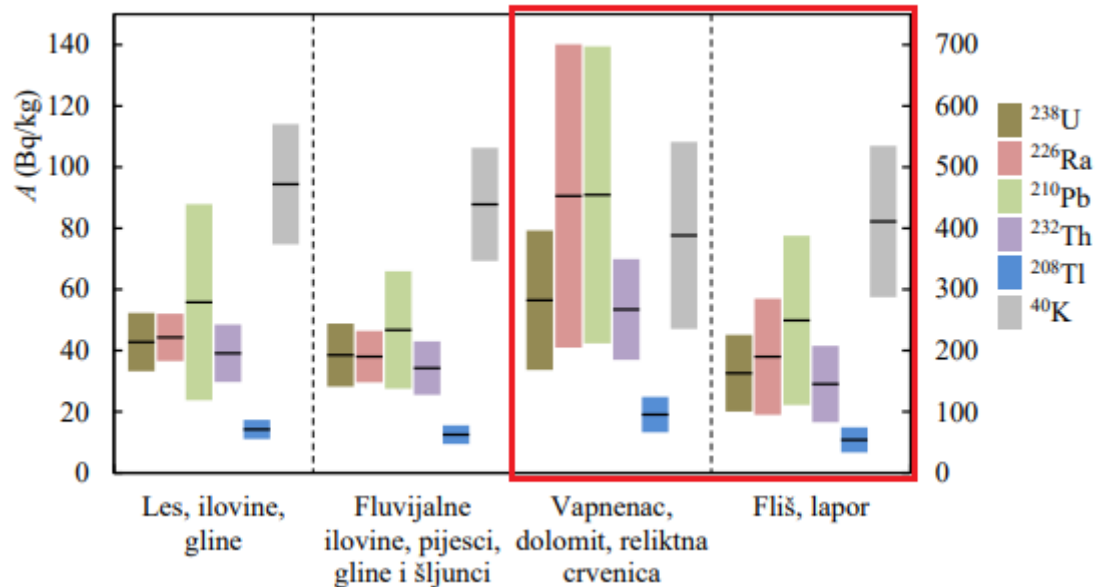
Slika 7. Koncentracije aktivnosti ( A ) u ovisnosti o matičnom supstratu tla. Vrijednosti A ^{40}\text{K} nekoliko puta su veće od ostalih vrijednosti pa se zbog bolje preglednosti lijeva vertikalna skala odnosi na ^{238}\text{U} , ^{226}\text{Ra} , ^{210}\text{Pb} , ^{232}\text{Th} i ^{208}\text{Tl} , a desna na ^{40}\text{K} (izvor: Šošćarić 2017)
