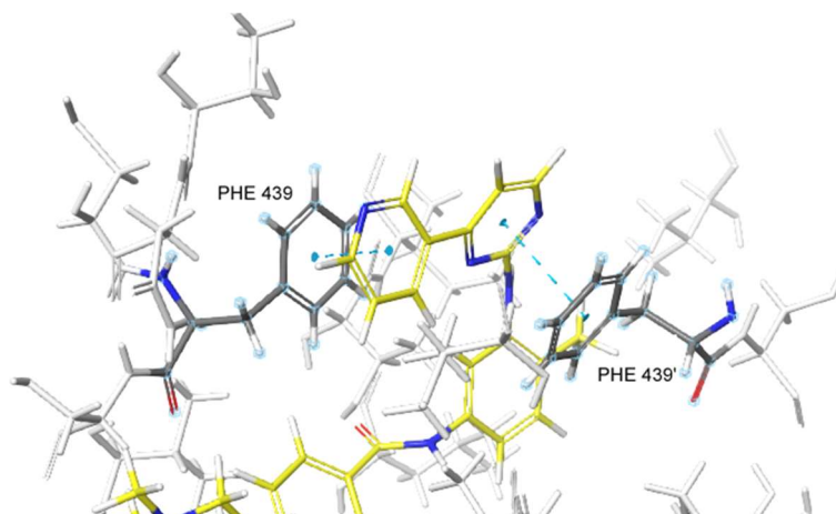
Slika 13. Nekovalentne interakcije liganda STI sa šupljinom 1. \pi - \pi interakcije naslagivanja između liganda STI (žuto) i bočnih ogranaka aminokiselina Phe 439 (sivo) označene su plavom isprekidanom linijom. Aminokiseline unutar šupljine 1 označene su bijelom bojom.
