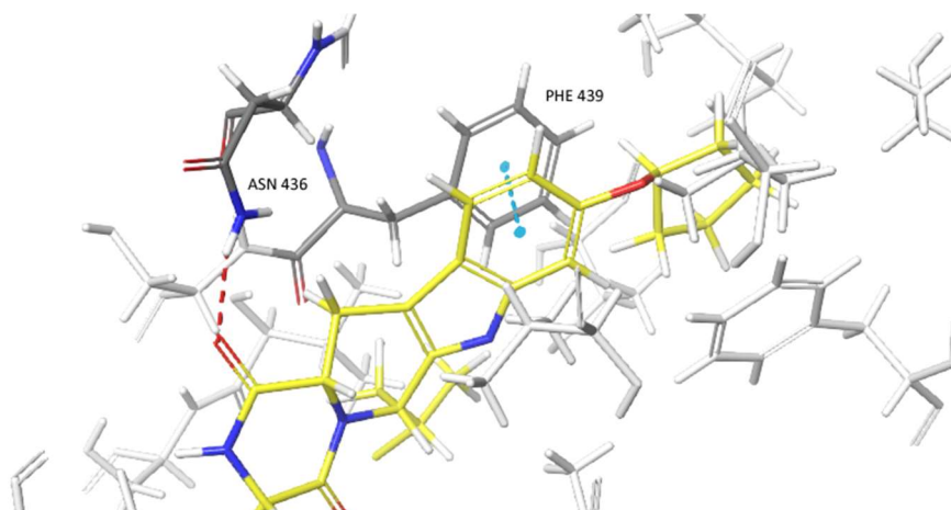
Slika 11. Nekovalentne interakcije liganda MZ29 sa šupljinom 1. \pi - \pi interakcije naslagivanja između liganda MZ29 (žuto) i bočnog ogranaka aminokiseline Phe 439 (sivo) označene su plavom isprekidanom linijom. Vodikova veza koju tvore kisik keto-skupine pirazinskog prstena liganda MZ29 te dušik aminokiseline Asn 436 (sivo) označena je crvenom isprekidanom linijom. Aminokiseline unutar šupljine 1 označene su bijelom bojom
