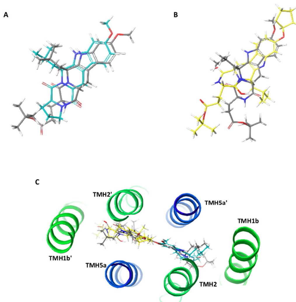
Slika 9. Vežanje liganada FTC , Ko143 te MZ29 u šupljini 1 proteina ABCG2: A) Preklapljenе strukture najboljeg načina vežanja liganada FTC (plavo) i liganada Ko143 (sivo) u šupljini 1. B) Preklapljenе strukture najboljeg načina vežanja liganada MZ29 (žuto) te drugog najboljeg načina vežanja liganada Ko143 s istim afinitetom vežanja koji se nalazi na suprotnoj strani šupljine 1 u odnosu na prvi način vežanja. C) Smještaj liganada FTC , Ko143 te MZ29 u unutrašnjosti transmembranske domene koju čine transmembranske zavojnice TMH2/TMH2', TMH5a/TMH5a' te TMH1b/TMH1b'.
