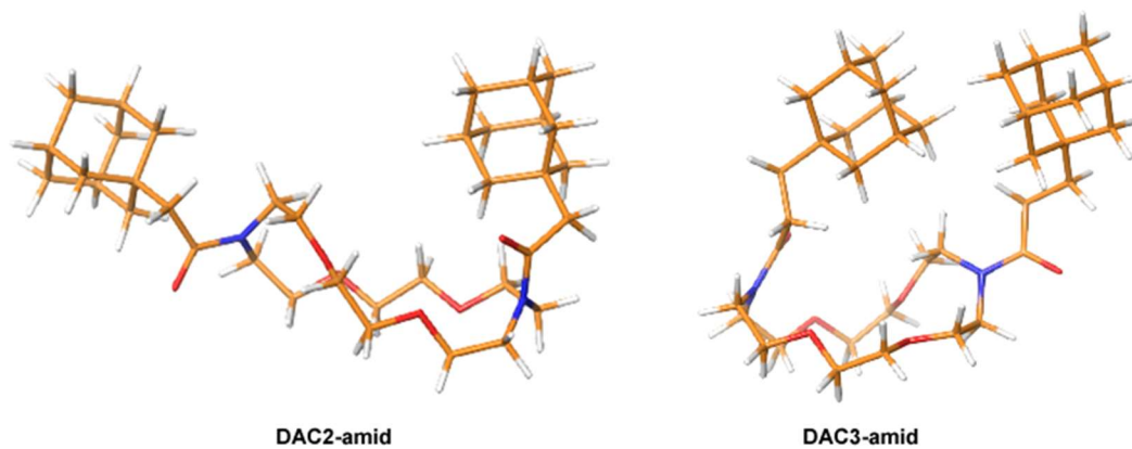
Slika 16. Konformeri DAC-amida dobiveni računima molekulskog uklapanja na protein ABCG2.
