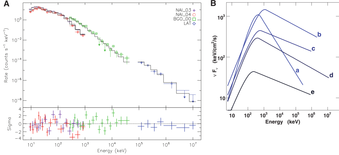
Slika 1.7: Spektar bljeska gama-zračenja GRB 080916C.
