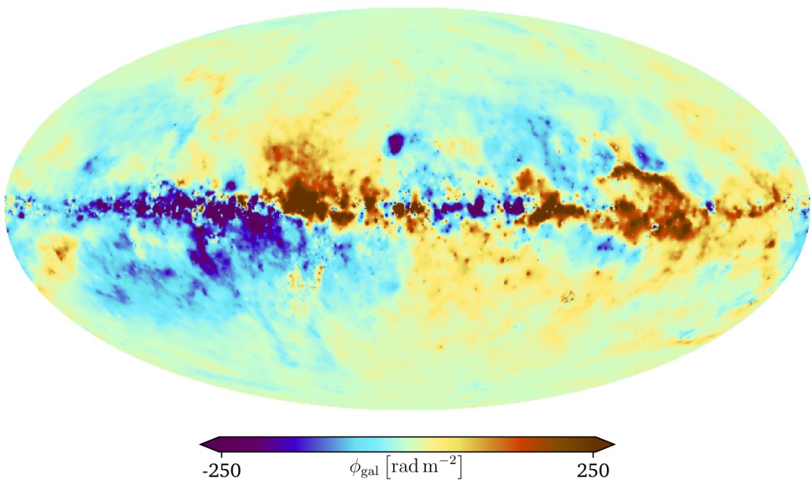
Slika 4.4. Karta ukupne galaktičke Faradayeve rotacije na cijelom nebu [22].
