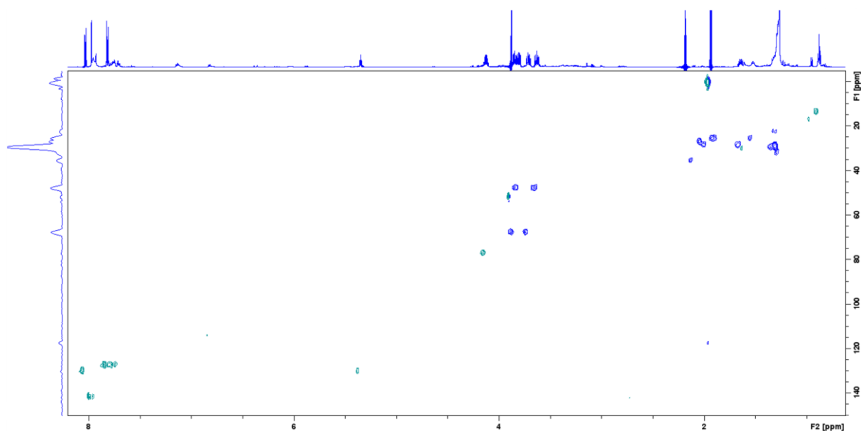
Slika D6. Spektar HSQC onečišćenja 3-16-c snimljen u CD 3 CN pri 25 °C.
