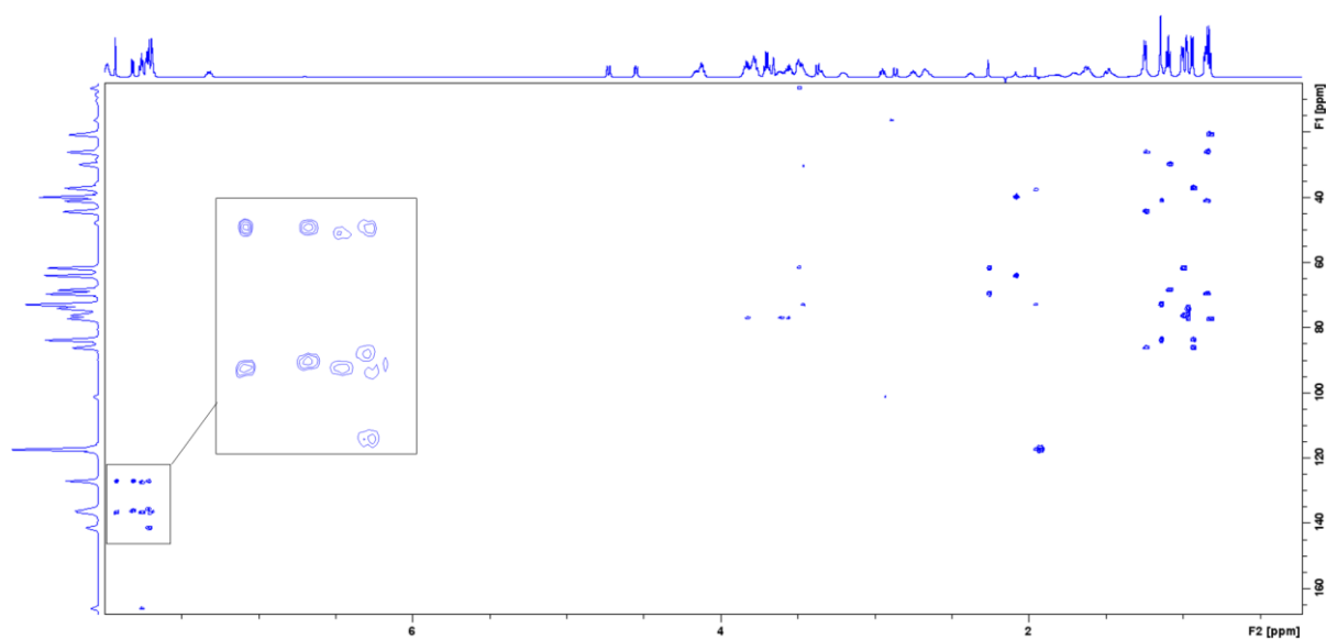
Slika D10. Spektar HMBC onečišćenja 3-16-i snimljen u \text{CD}_3\text{CN} pri 25\text{ }^\circ\text{C} .
