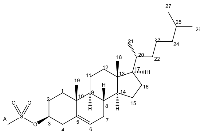
Slika 28. Strukturna formula spoja 6
