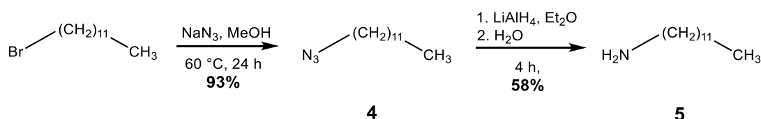
Slika 41. Shematski prikaz pripreve dodecilnog prekursora 5
