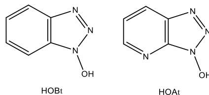
Slika 14. Strukturne formule najčešće korištenih aditiva
