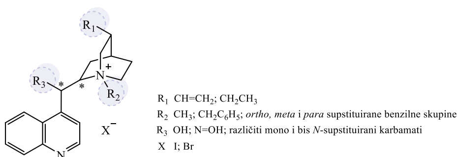
Slika 2. Opće strukturne formule sintetiziranih spojeva, derivata cinhonidina (8 S , 9 R ) i cinhonina (8 R , 9 S ).
