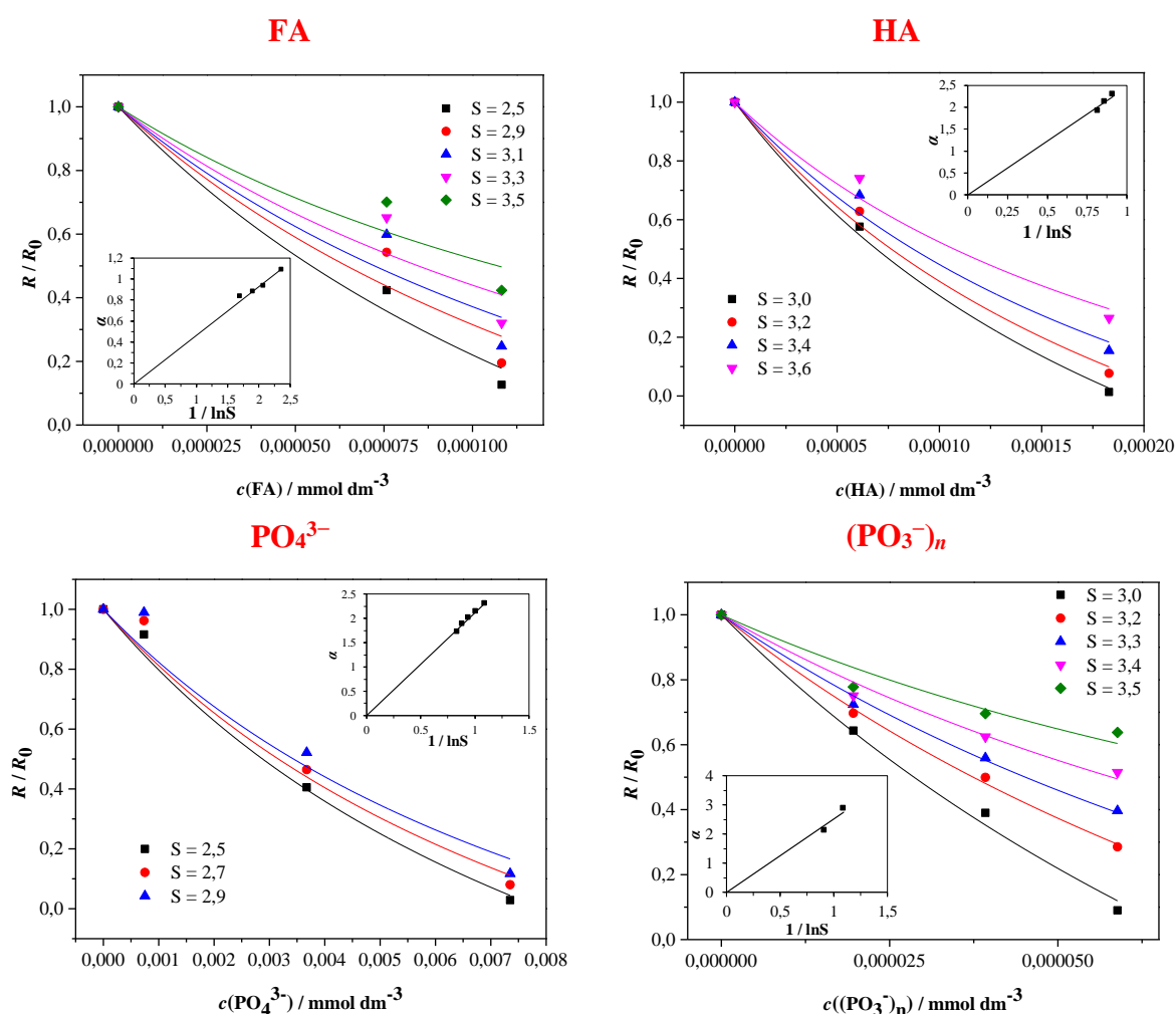
Slika 4.55. Relativna brzina rasta kristalnog sjemena kalcita u ovisnosti o koncentraciji dodanih aditiva pri \theta = 20^\circ\text{C} i masenoj koncentraciji kristala romboedarskog kalcita \gamma(\text{kalcit}) = 0,250\text{ g dm}^{-3} te prezasićenostima naznačenim na slici. FA – fulvinska kiselina, HA – huminska kiselina, PO_4^{3-} – fosfatni ioni i (PO_3^-)_n – polifosfatni ioni.
