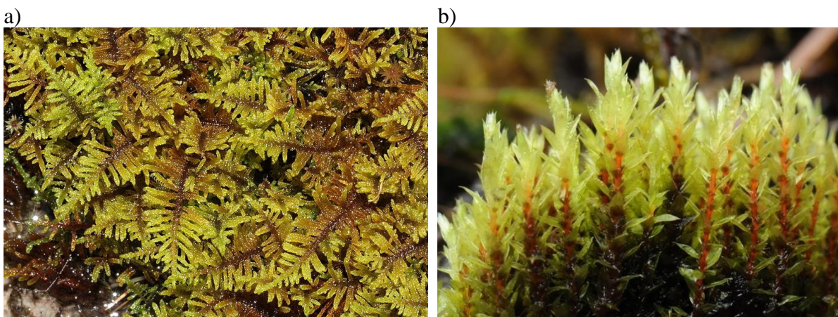
Slika 2.10. Mahovine koje sudjeluju u izgradnji dva tipa sedrenih makrostruktura: a) Palustriella commutata , prema referenci 37; b) Ptychostomum pseudotriquetrum , prema referenci 38.
