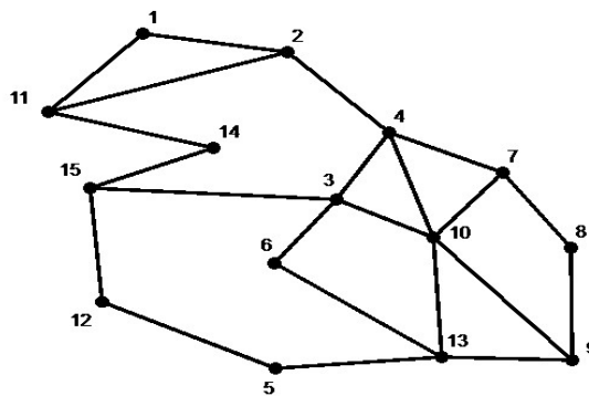
Slika 4.4: Javni ključ
