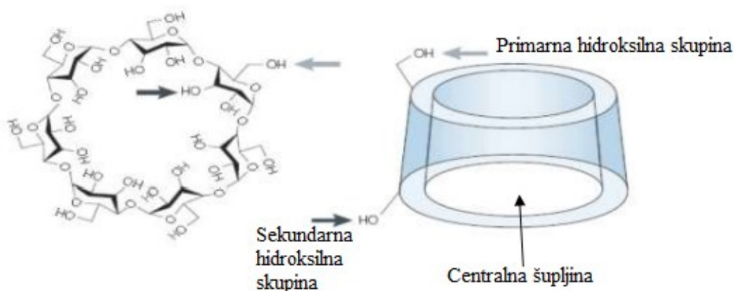
Slika 10. Struktura \beta -ciklodekstrina te prikaz oblika krnjeg stošca (preuzeto i prilagođeno iz ref. 9).
