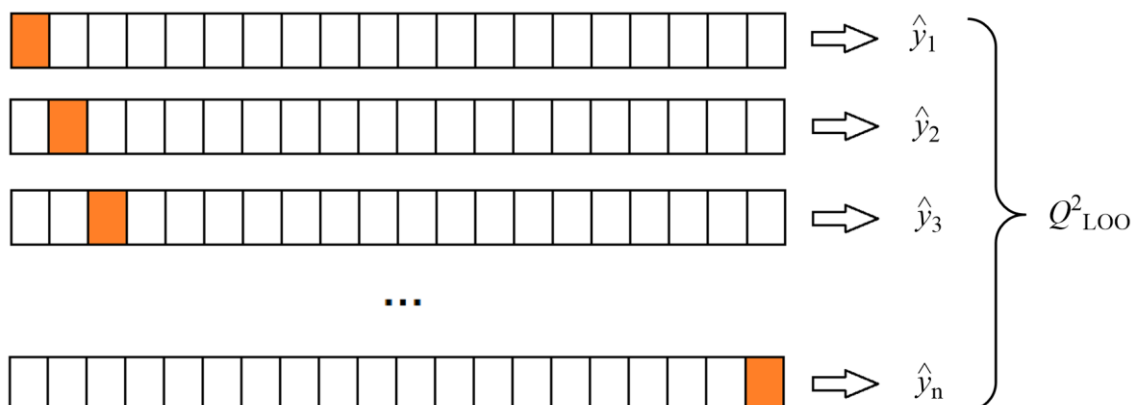
Slika 1. Shematski prikaz LOO unakrsne validacije. Iz trening skupa iterativno se izostavlja po jedan spoj i predviđa mu se aktivnost modelom razvijenim na preostalim spojevima.
