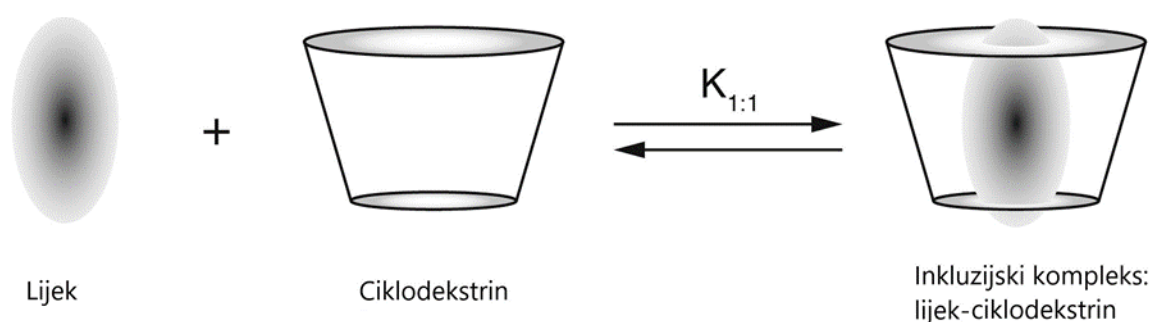
Slika 4. Tvorba inkluzijskog kompleksa lijeka i ciklodekstrina u omjeru 1:1
