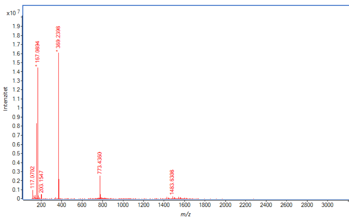
Slika 44. Spektar masa otopine cinarizina s HP \beta CD ( c = 4,40 \cdot 10^{-5} \text{ mol dm}^{-3} ) u sustavu otapala metanol:voda = 1:1. Ionizacija ESI+, napon fragmentora 50,0 V
