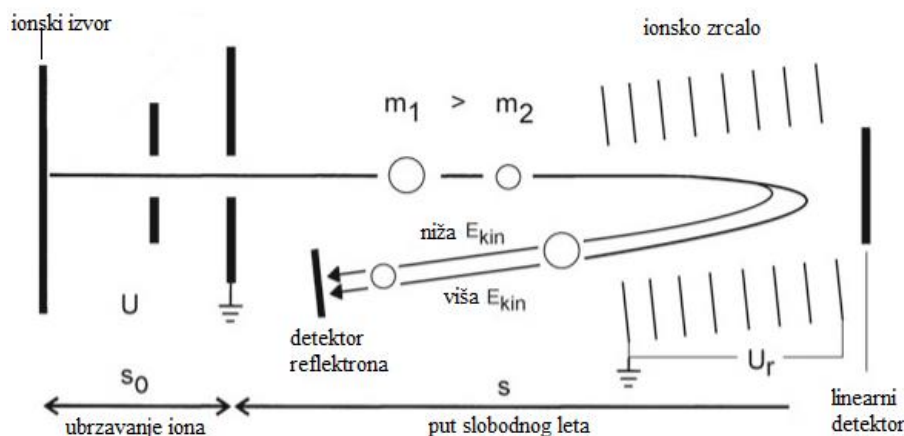
Slika 8. Shematski prikaz analize iona analizatorom masa koji mjeri vrijeme leta s ionskim zrcalom. E_{kin} označava kinetičku energiju, U označava početni napon kojim se ubrzavaju ioni, a U_r napon koji se primjenjuje u ionskom zrcalu
