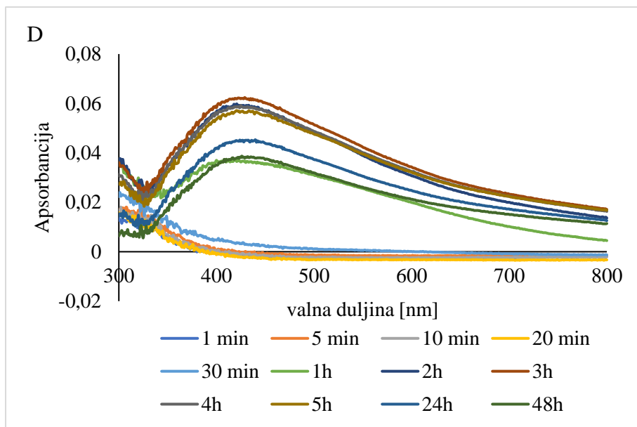
Slika 3. Apsorpcijski spektri AgNO 3 koncentracije 1,5 mg/L u A) ultračistoj vodi s dodatkom 1 %-tne glukoze, B) BBM podlozi s dodatkom 1 %-tne glukoze, C) ultračistoj vodi bez dodatka glukoze i D) BBM podlozi bez dodatka glukoze. Spektri su dobiveni mjerenjem apsorbancije uzoraka u rasponu valnih duljina od 300 do 800 nm u vremenskim intervalima od 0, 1, 5, 10, 20 i 30 minuta te 1, 2, 3, 4, 5, 24 i 48 sati.
